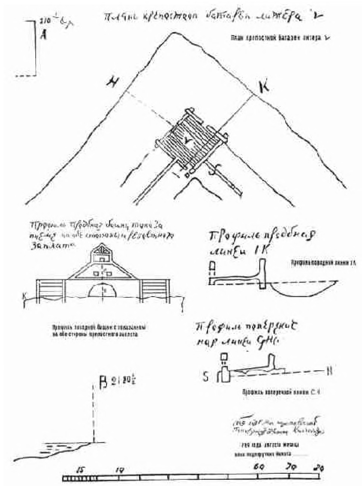
Рис. 7: Инженерный разрез бастионов Табынской крепости 1736 г.
